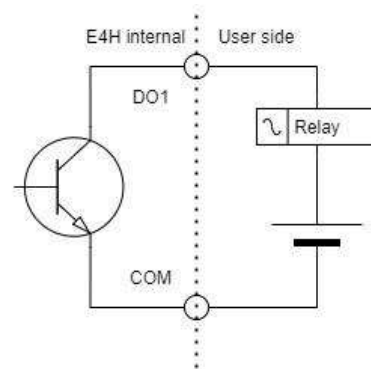
[그림6] DO 사용 예
