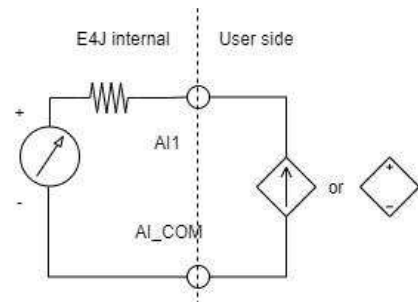
[그림7] AI의 내부 회로 모델과 사용 예
