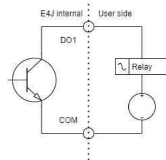
[그림6] DO의 내부 회로 모델과 사용 예
